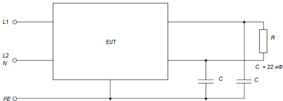
Рисунок I.1 – Испытательная цепь для измерения изменения эталонного (опорного) потенциала, вызванного нагрузкой – однофазный выход
